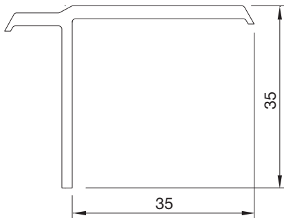
PTS3160BY.0003 ASİMETRİK T T COVERING
