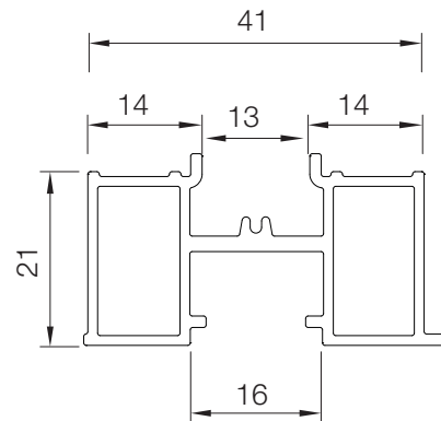
İSPANYOLET YÜKSELTME PROFİLİ ESPAGNOLETTE UPGRADE PROFILE
